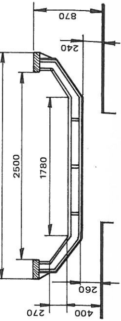
Snit (Skala 1:50)
